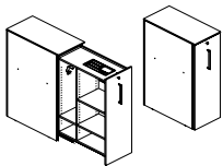
Caisson haut L40 x P80 x H110,7 cm Structure mélaminé Blanc (BL) ou Noir (MK) Poignée Aluminium (AF), Blanc (BW) ou Noir (NF) À compléter d'un top
