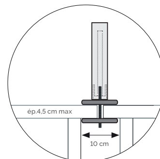
3 - Étrier double plateau ép. 4.5 max
